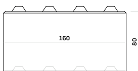
PROSPETTO
